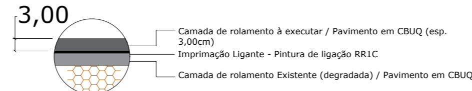
DETALHE PAVIMENTAÇÃO Escala 1:10
