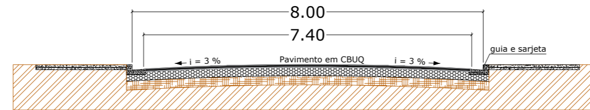
CORTE LONGITUDINAL RECAPEAMENTO Escala 1:100
